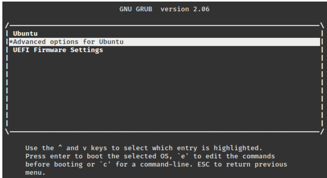
Fig. 1: Grub Menu
