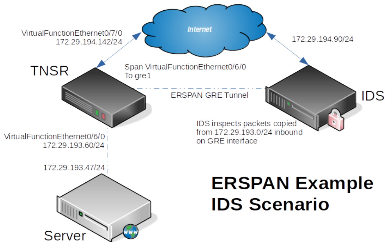
Fig. 7: ERSPAN Example
